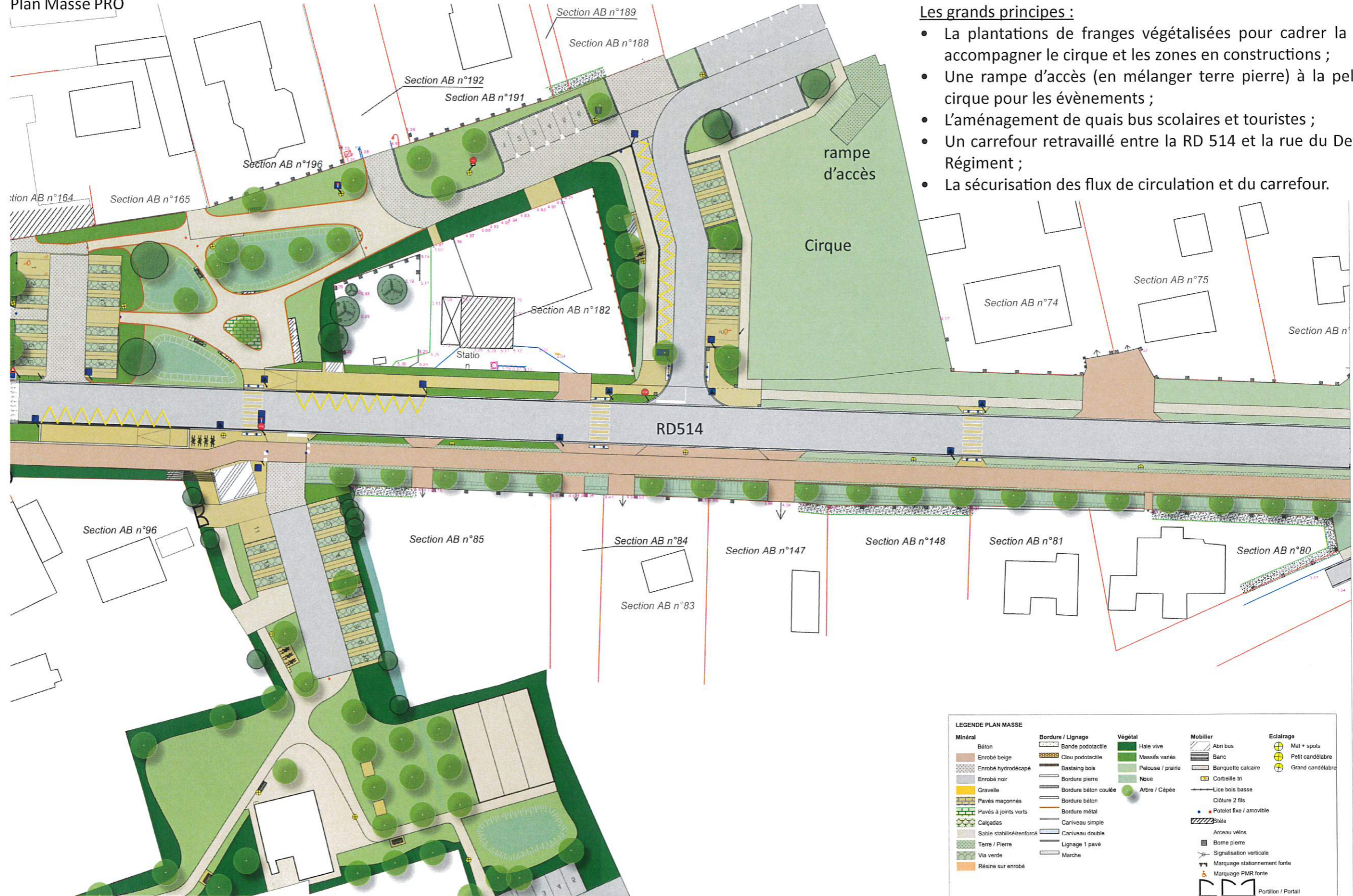
Plan Masse PRO
